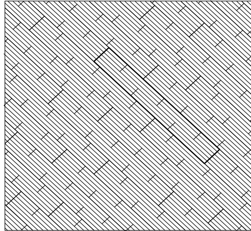
LHP Ungeordneter Verband diagonal
